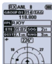
Wegpunkt-NAV-Display
